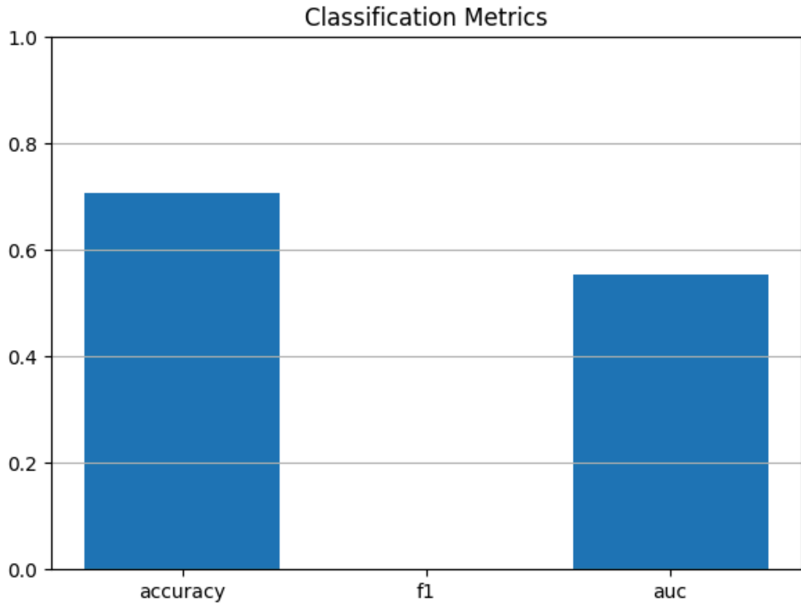
classification_metrics_bar_chart.png
